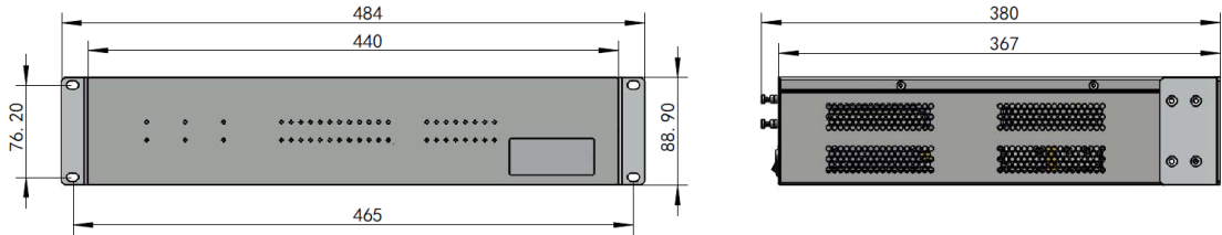
图 2-1 尺寸图
