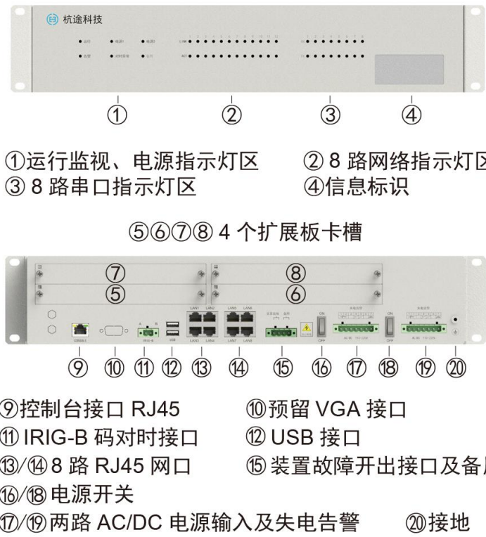
图 2-2 接口说明图
