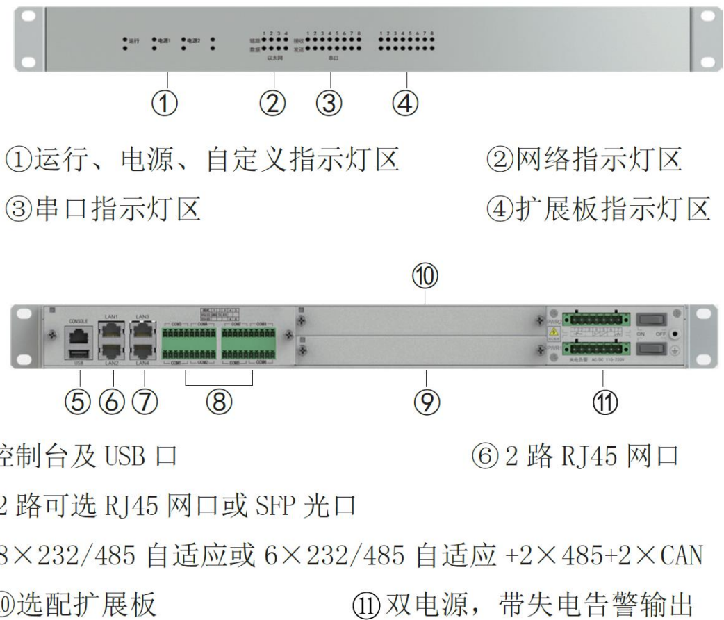
图 2-1 接口示意图
