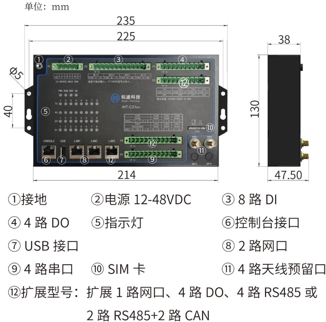
图 2-1 iHT-C31F 尺寸及接口说明图
