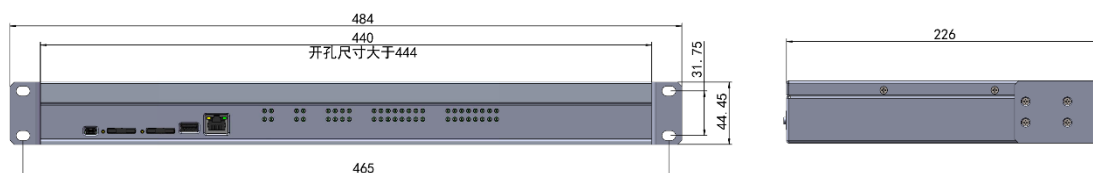
图 2-4 安装方式及尺寸示意图
